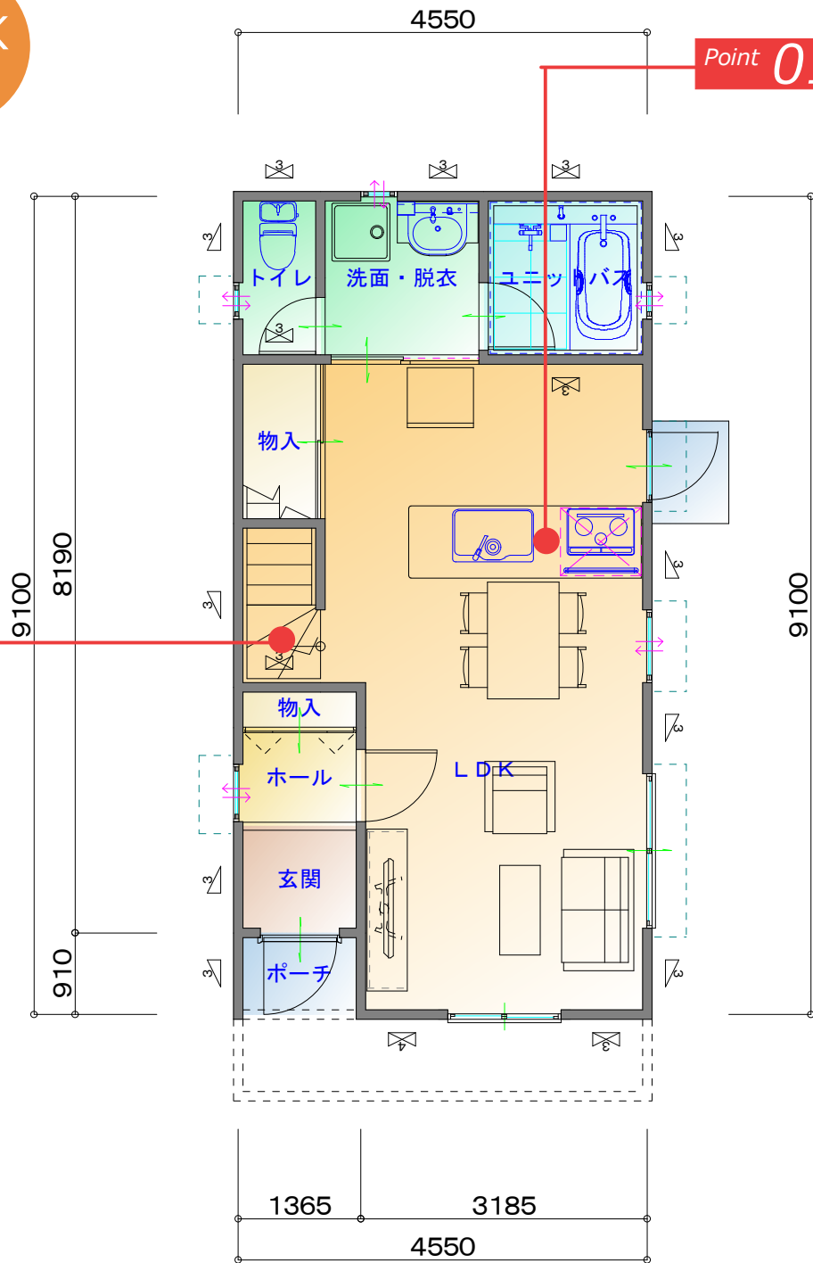
1F 平面図
