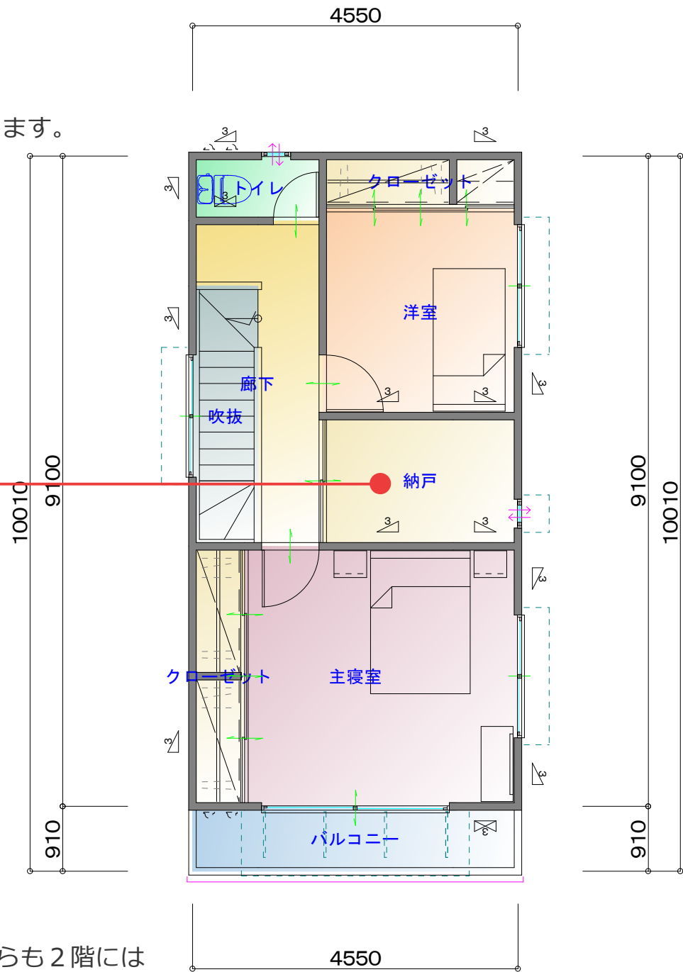
2F 平面図
