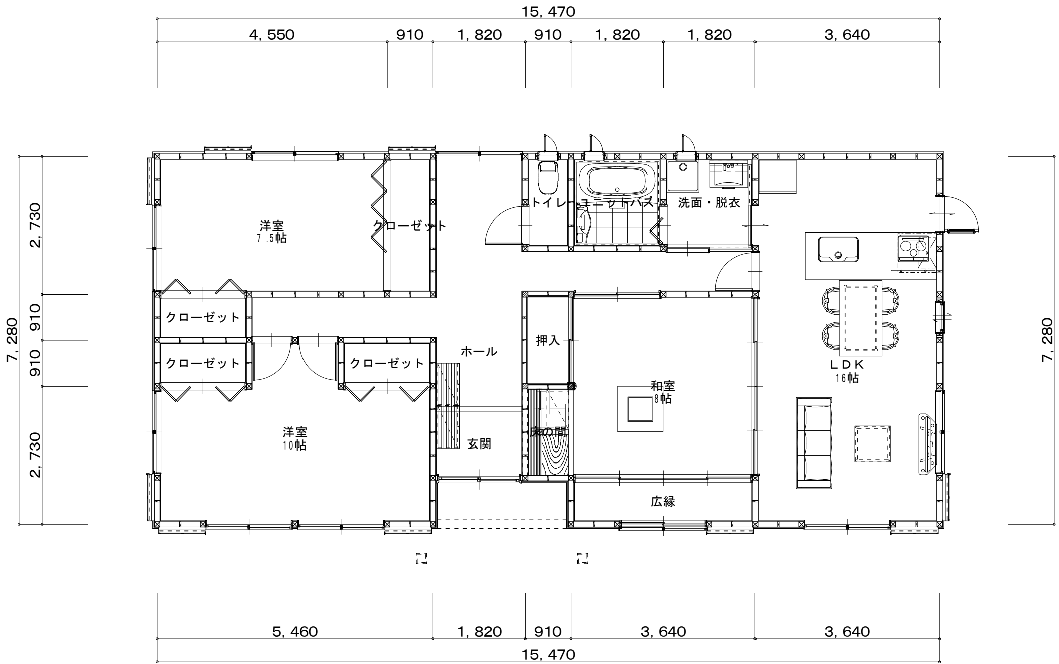
平面詳細図 1階
