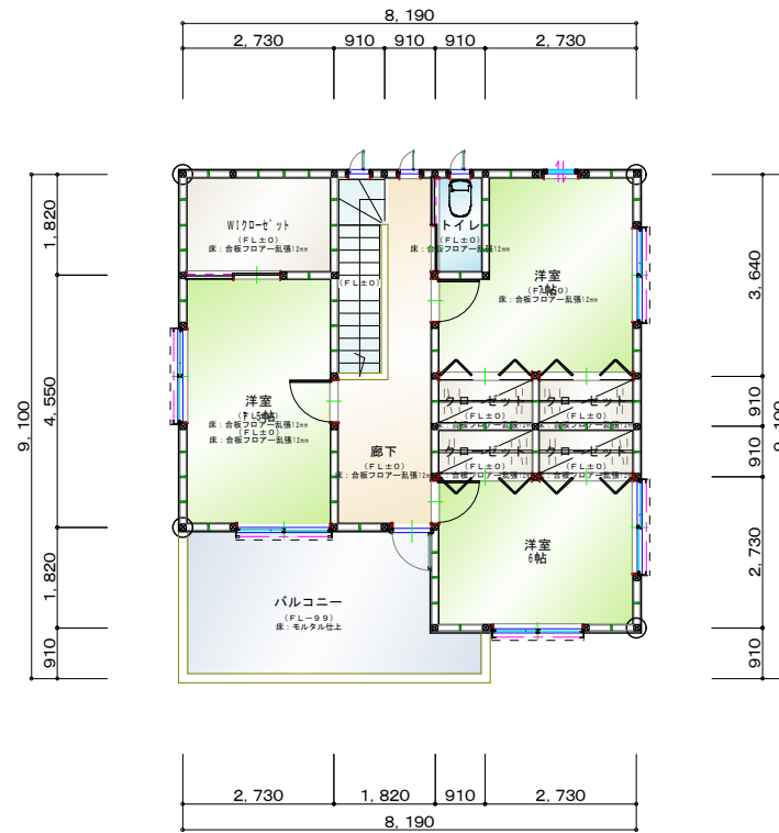
平面詳細図 2階
