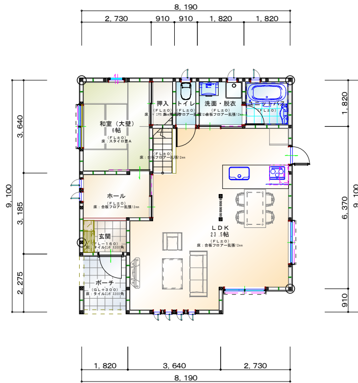
平面詳細図 1階
