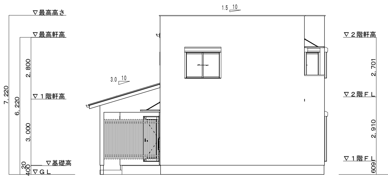
西側立面図
