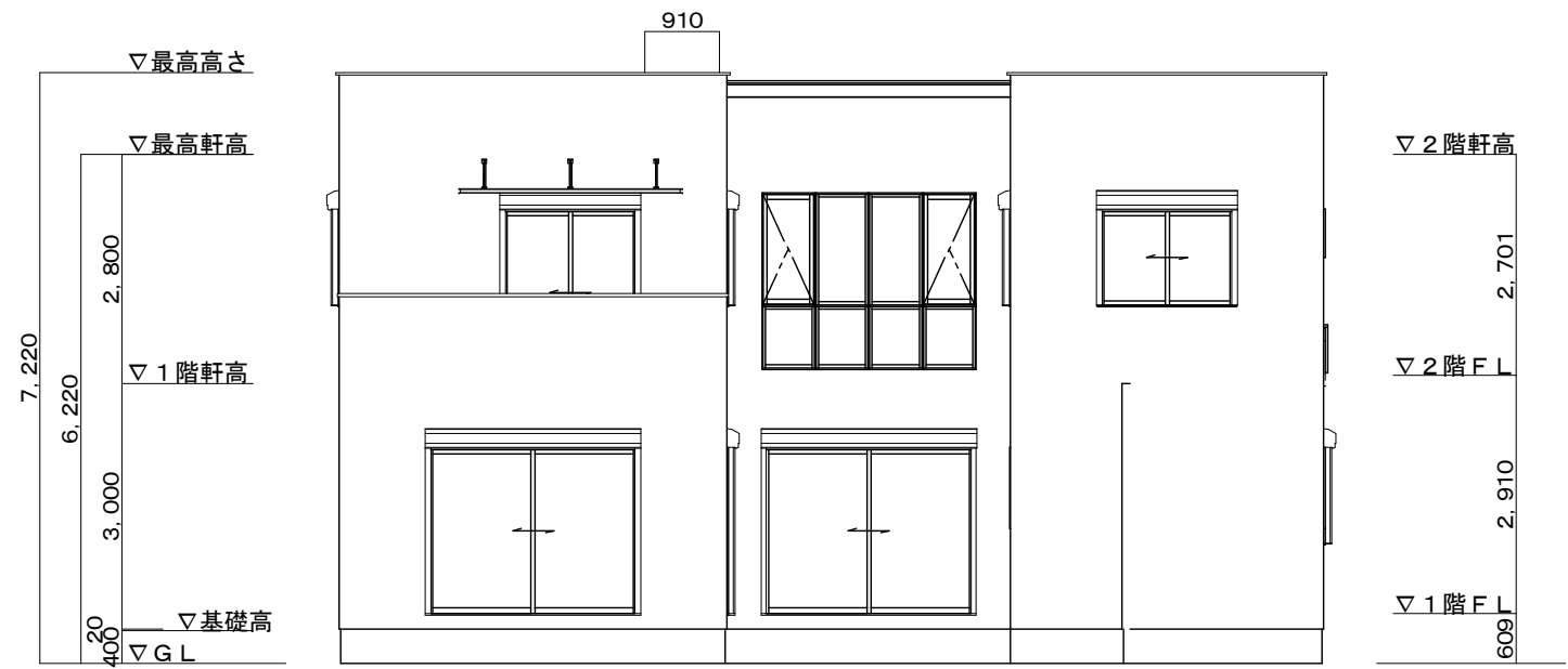
南側立面図
