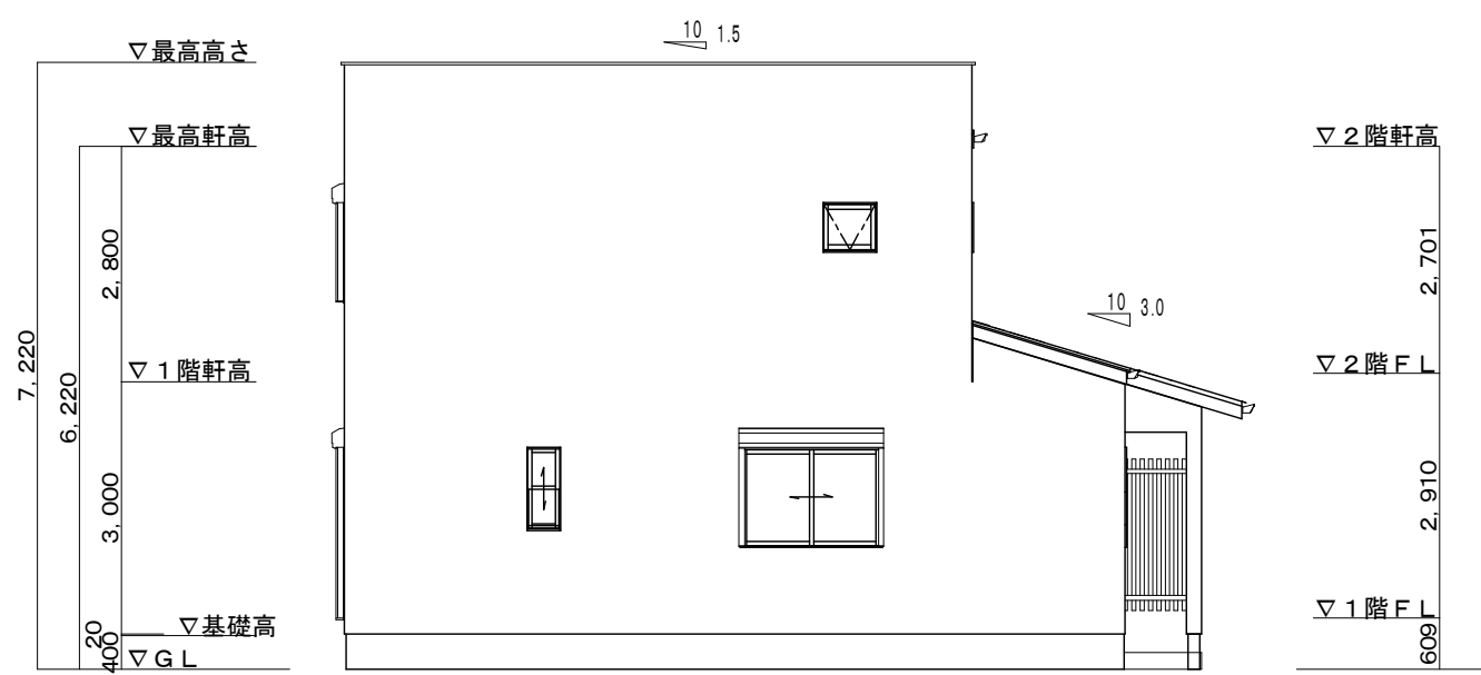
東側立面図
