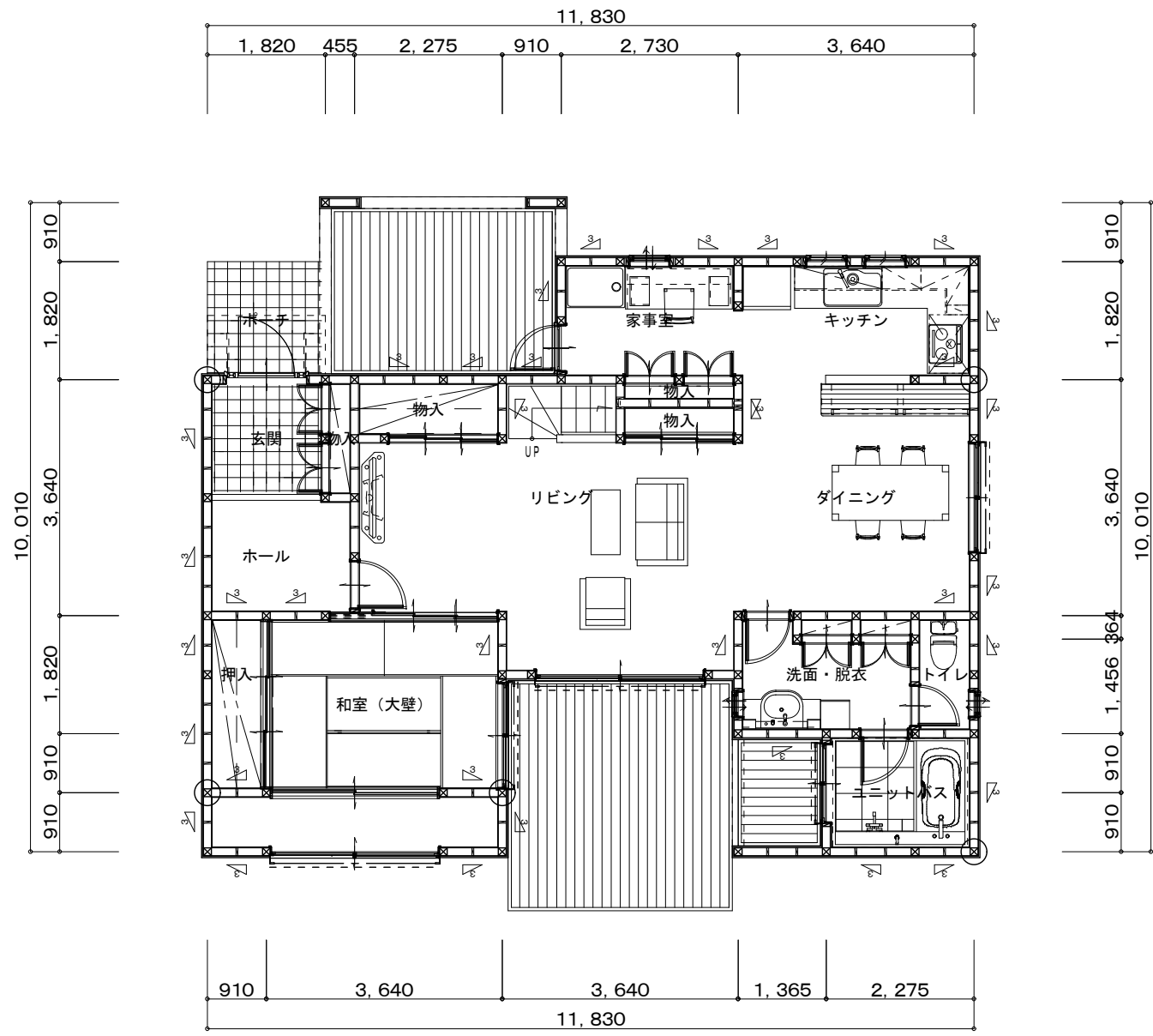
平面詳細図 1階
