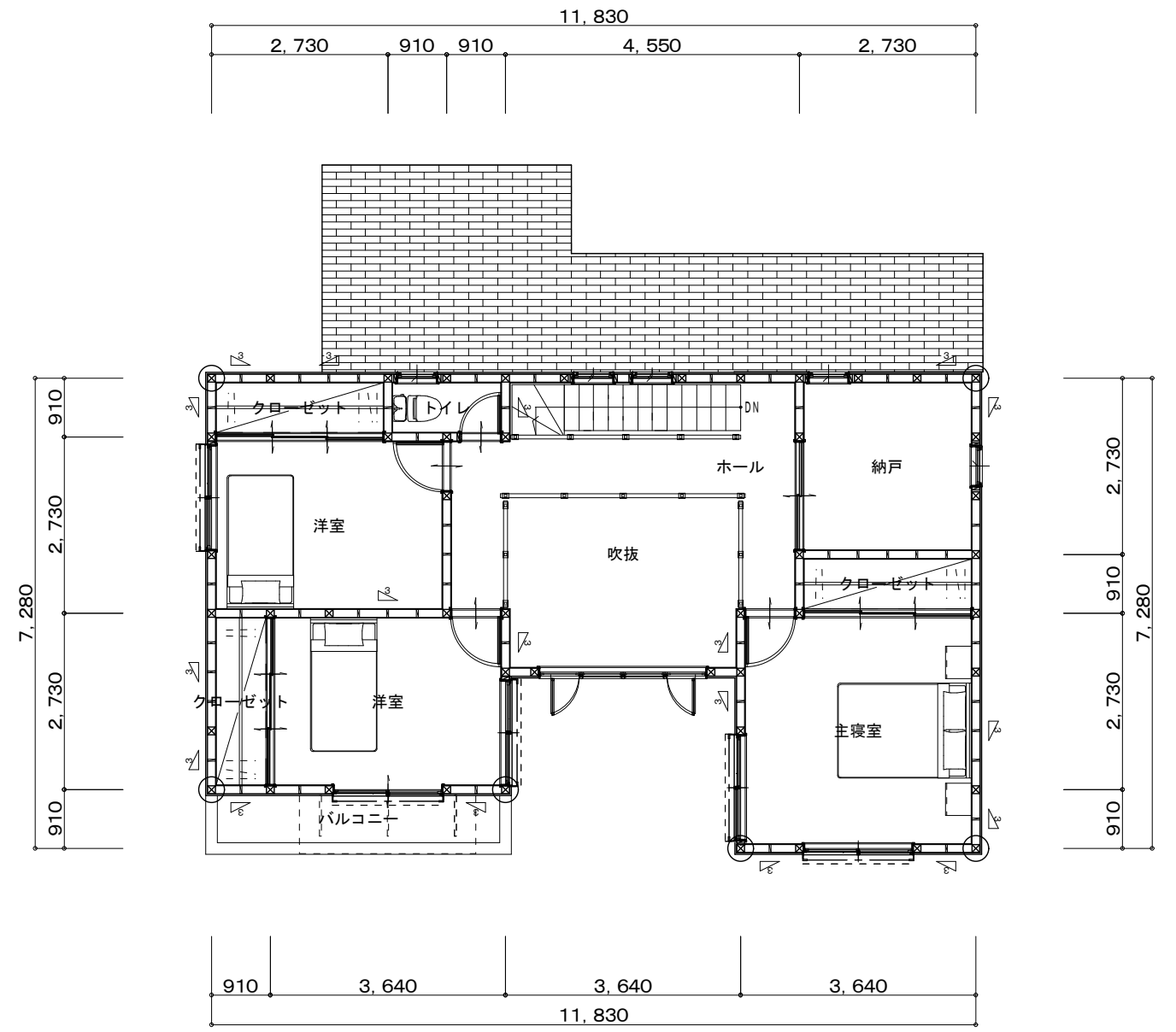
平面詳細図 2階
