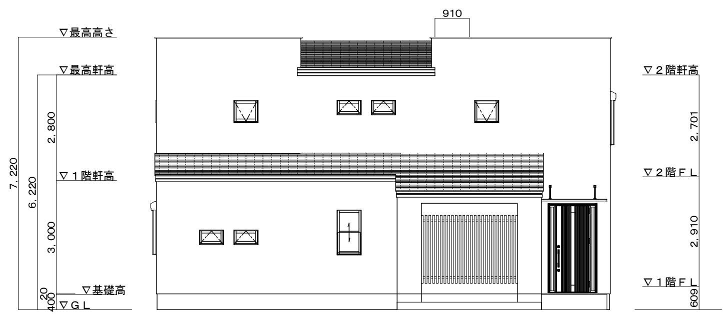
北側立面図
