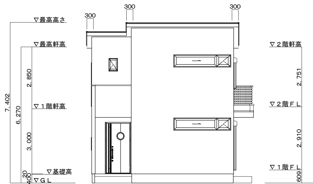
西側立面図
