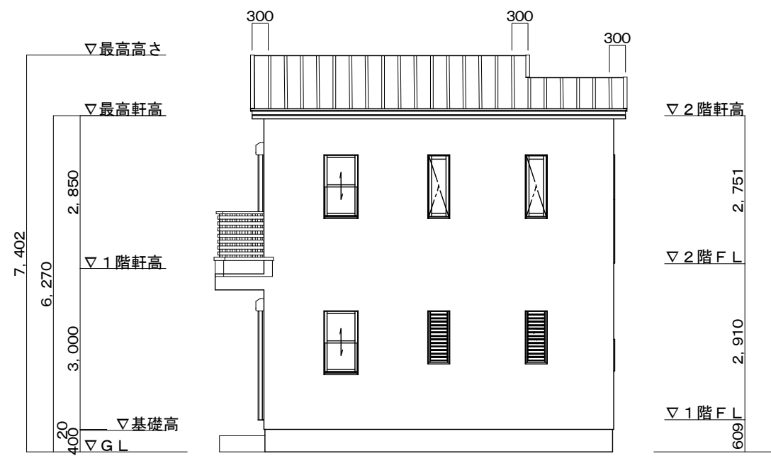
東側立面図
