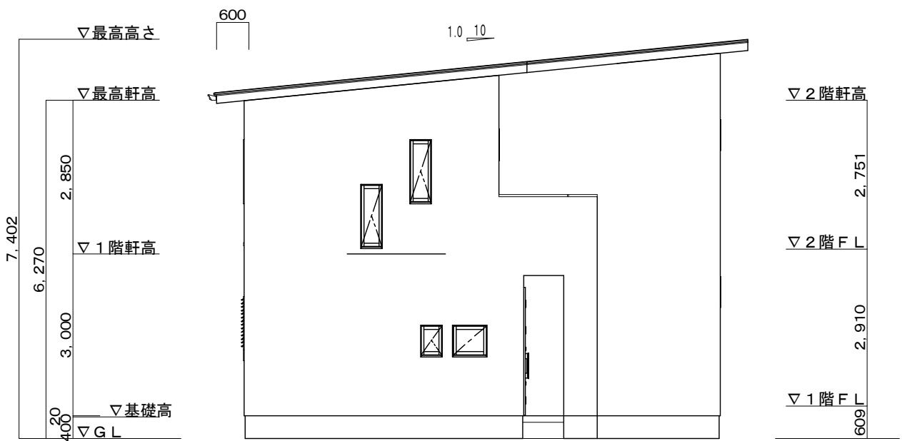
北側立面図
